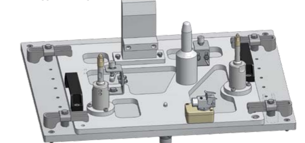
Posaggio a formato per il componente da trattare.
